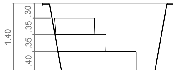
CORTE A
