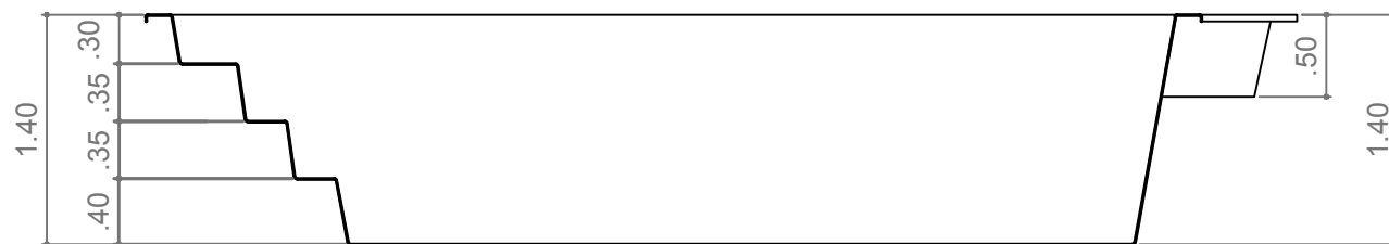
CORTE B
