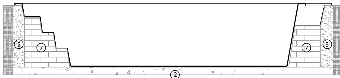
CORTE B
