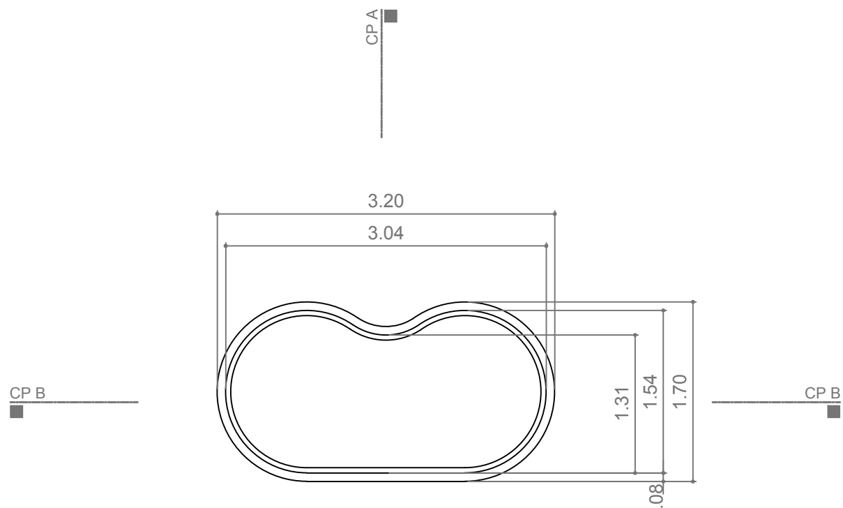
PLANTA BAIXA
