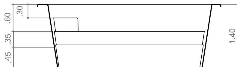
CORTE A
