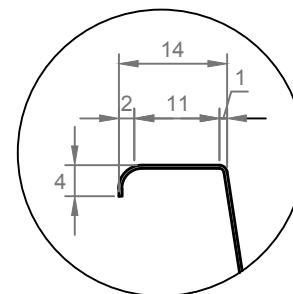
DETALHE BORDA SIMPLES
