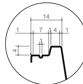
DETALHE BORDA REBAIXADA
