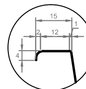
DETALHE BORDA SIMPLES
