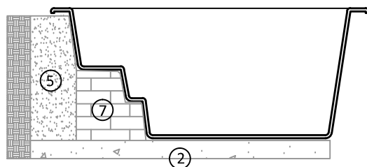
CORTE B
