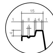
DETALHE BORDA REBAIXADA
