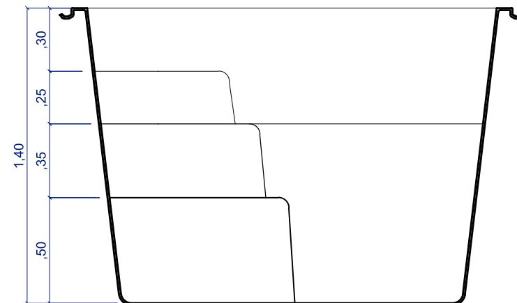
CORTE B 1:25
