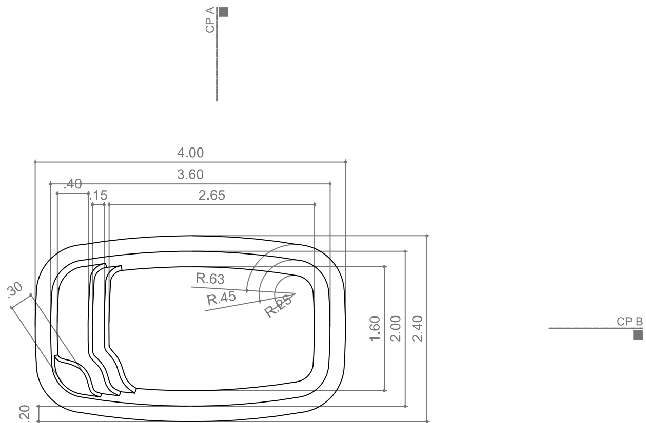
PLANTA BAIXA
