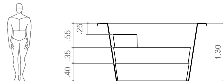
CORTE A
