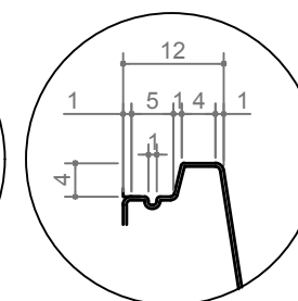
DETALHE BORDA REBAIXADA
