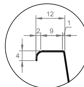
DETALHE BORDA SIMPLES
