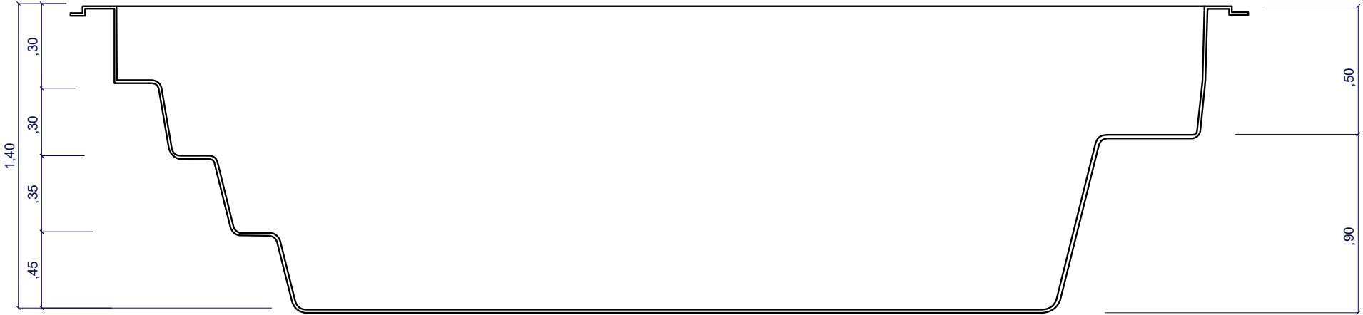
CORTE A 1:25
