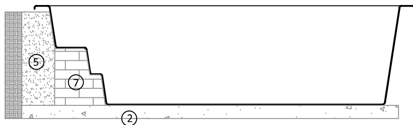
CORTE B
