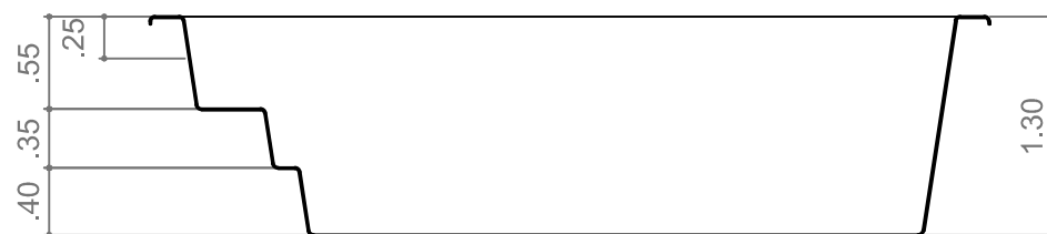
CORTE B
